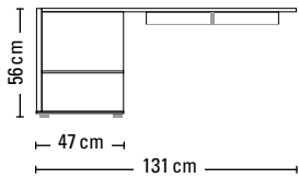
Anbau-Element links Nr. 854 für Schränke 850/851
