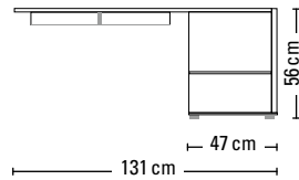
Anbau-Element rechts Nr. 855 für Schränke 850/851
