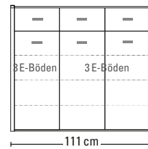
Schrank Nr. 1280
