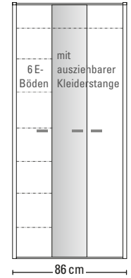
Spiegelschrank Nr. 1460
