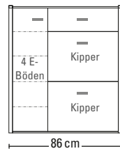
Schrank Nr. 1270
